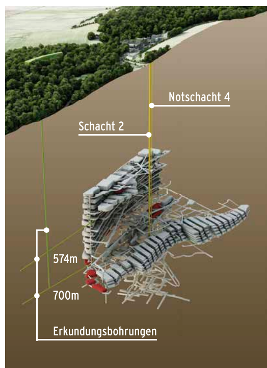
DIE WEGE DES ABFALLS: DER NEUE SCHACHT SOLL IN 574 UND 700 METER TIEFE MIT DEM BERGWERK VERBUNDEN WERDEN
